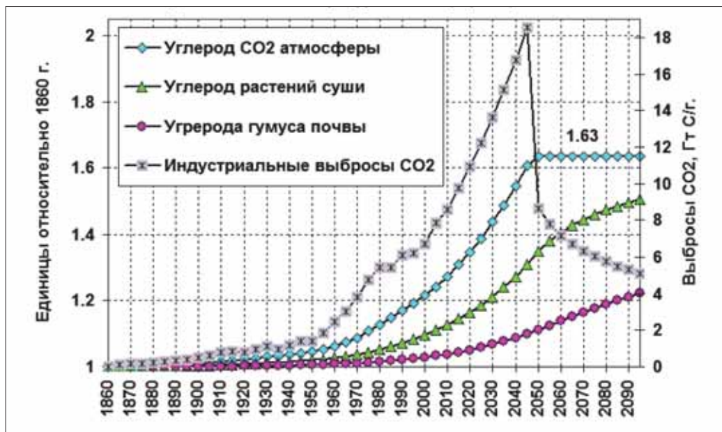
Рис. 13. Расчет оптимального управления. Концентрация \text{CO}_2 остается постоянной после достижения критической температуры 1,5^\circ \text{C} из Парижского соглашения. Представлены значения выбросов \text{CO}_2 , углерода в фитомассе лесов и органическом веществе почв. Координатная ось выбросов \text{CO}_2 находится справа.
