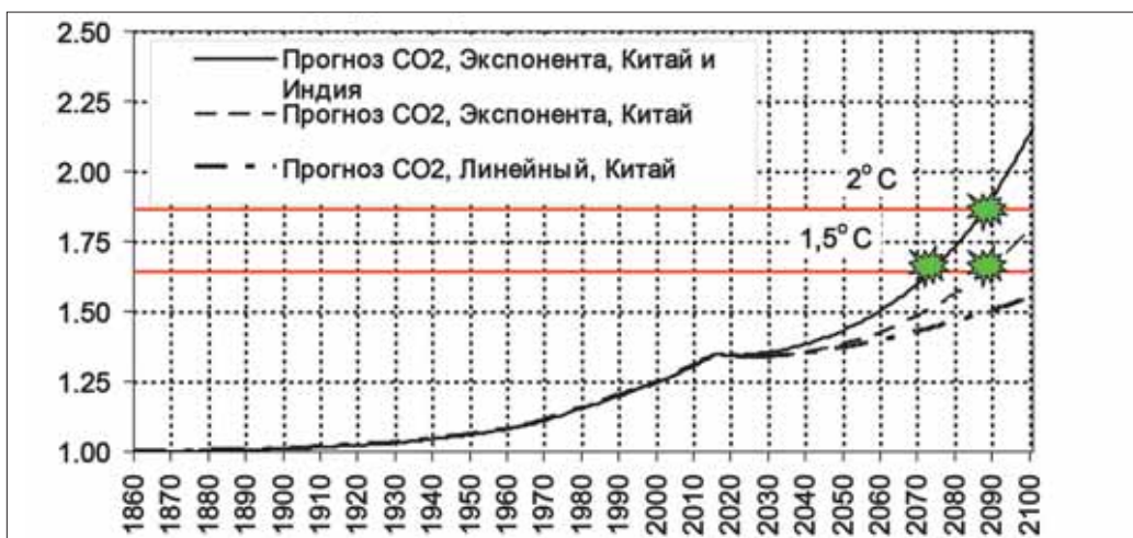
Рис. 12. Прогнозы относительного роста концентрации \text{CO}_2 в 1860-2100 г. После 2016 г. предполагается, что есть выбросы только Китая и Индии или Китая. Отмечены моменты достижения кривыми концентрации \text{CO}_2 значений, соответствующих прохождению через температуру атмосферы 1,5° и 2° C.
