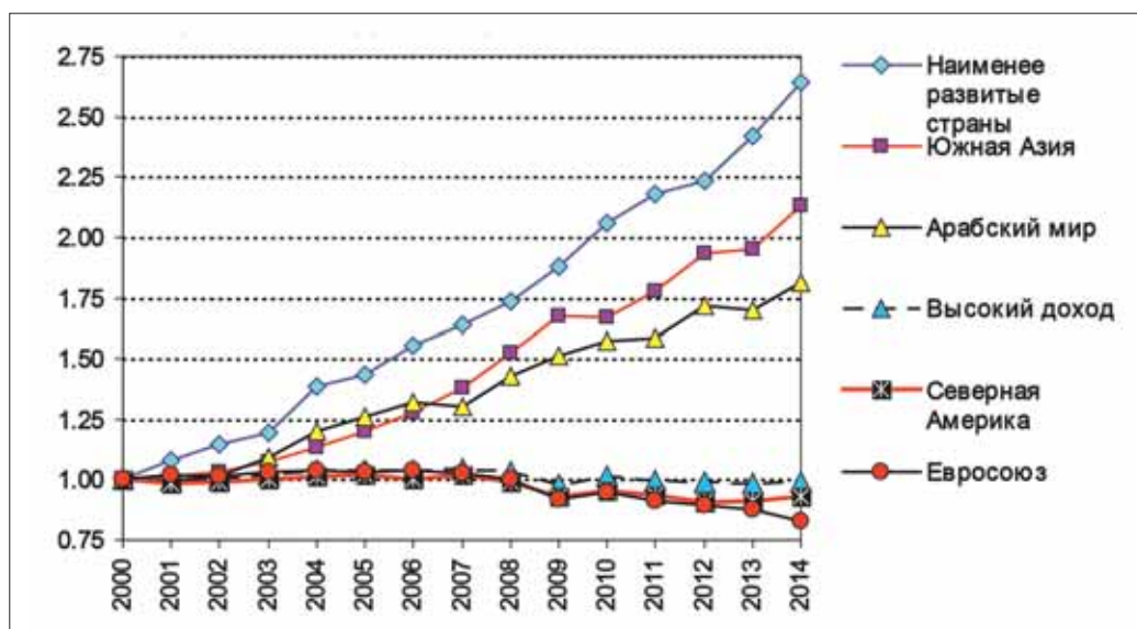
Рис. 8. Выбросы \text{CO}_2 в группах стран в 2000–2014 гг.
