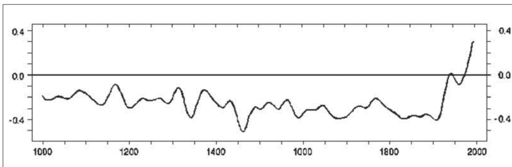
Рис. 7 Динамика средней глобальной температуры атмосферы ( ^{\circ}\text{C} ) за последнее тысячелетие по данным МГЭИК. По горизонтальной оси – годы, н.э.
