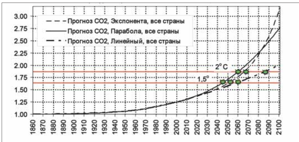
Рис. 11. Прогнозы относительного роста концентрации \text{CO}_2 в 1860-2100 г. После 2016 г. рост выбросов каждой страны задан указанной линией регрессии. Отмечены моменты достижения кривыми концентрации \text{CO}_2 значений, соответствующих прохождению через температуру атмосферы 1,50 и 2° C.
