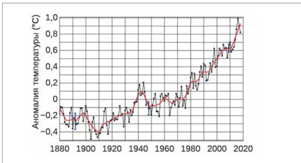
Рис. 6. Изменение глобальной температуры атмосферы в 1880-2019 гг. Сглаженная линия – пятилетние скользящие средние значения. Данные ВМО (Всемирная метеорологическая организация).
